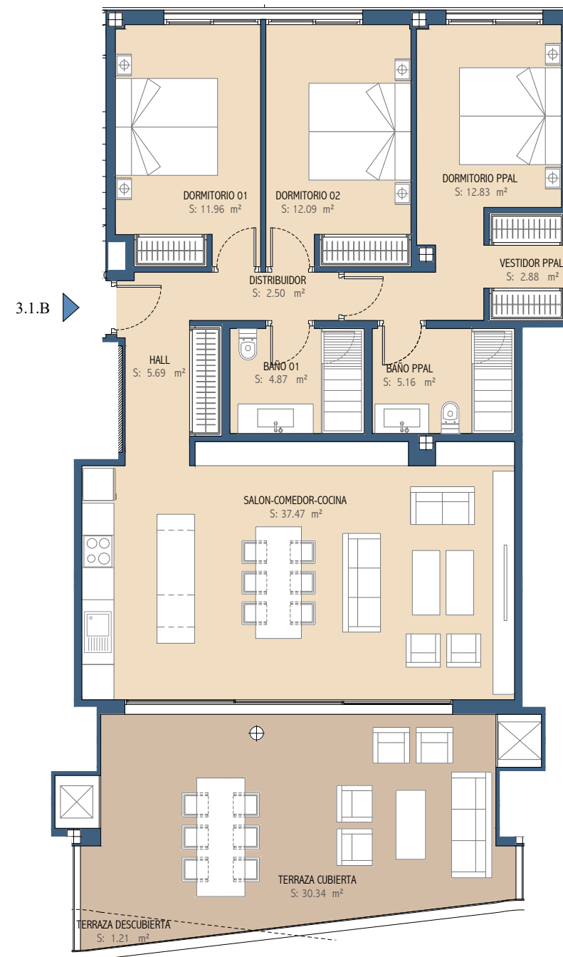
PLANTA PRIMERA
